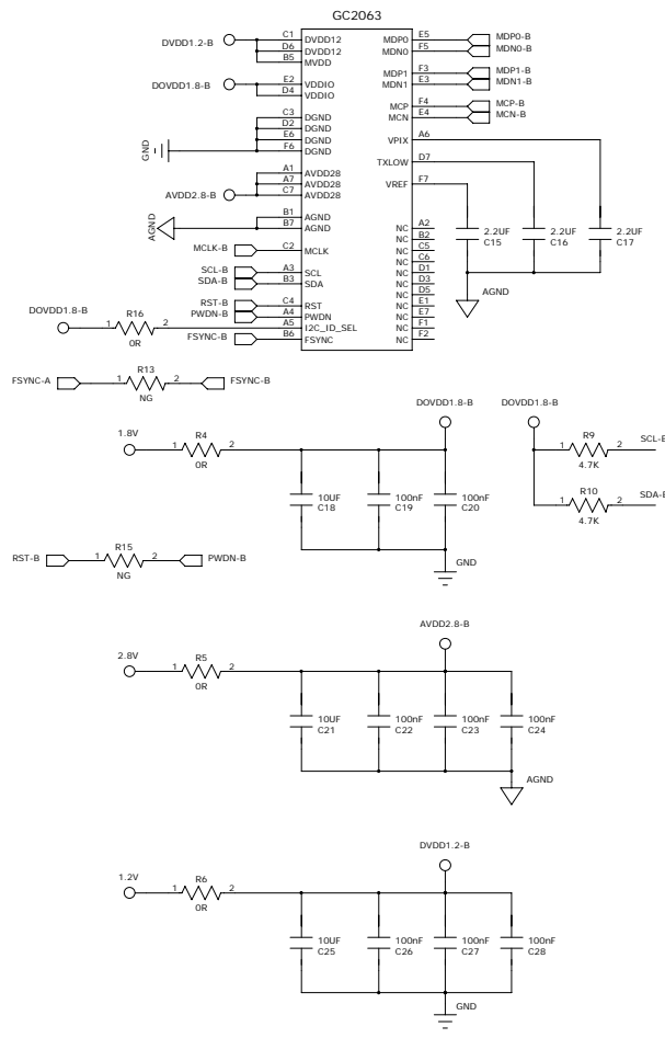
图 2-2 MIPI 接口 (2 lane) 外围电路
